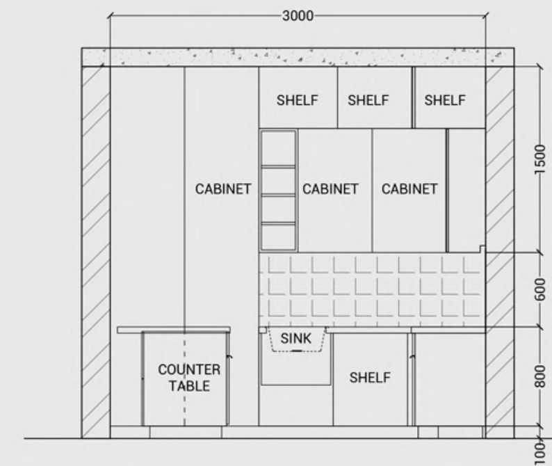
ELEVATION BB'
