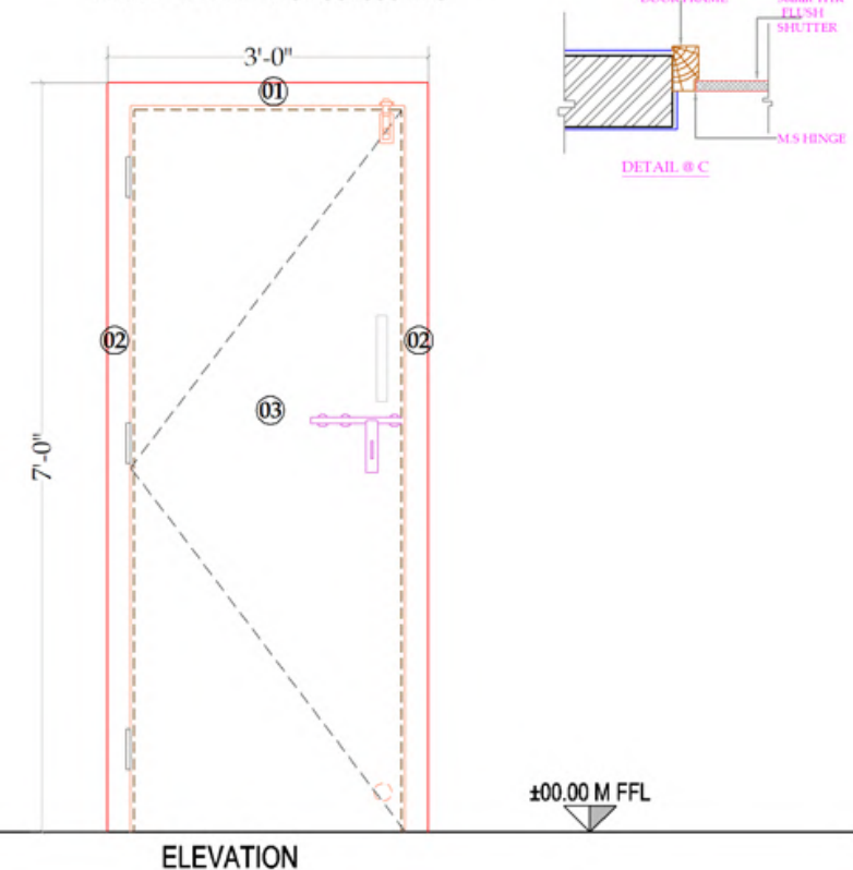
D1 - 3'0"X7'0" 06 NO'S
