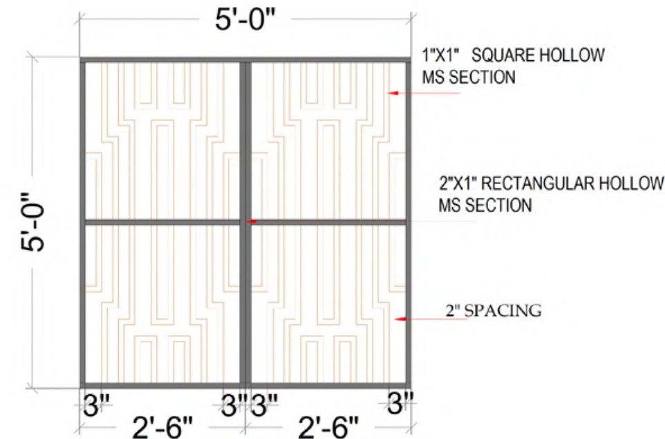
ELEVATION - 2 NOS
