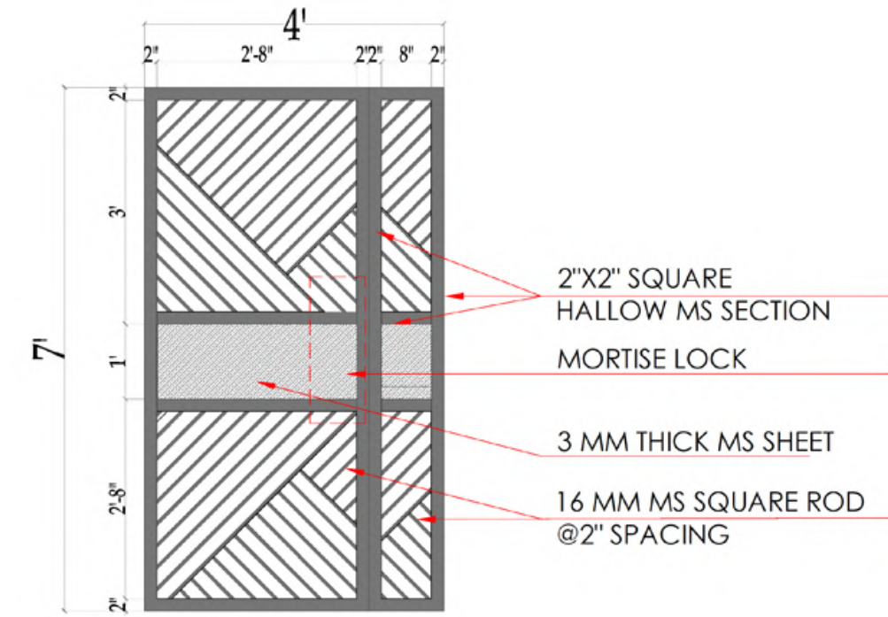
DOOR ELEVATION
